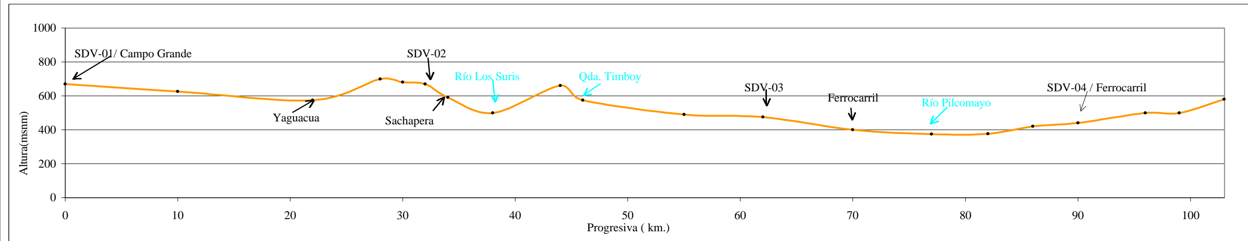
Perfil longitudinal de la sección; progresiva 0-100
