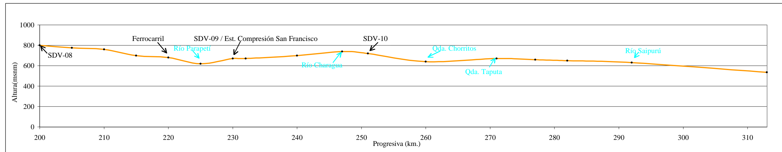
Perfil longitudinal de la sección; progresiva 200-300
